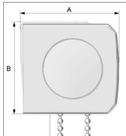
S2: Dimensions A: 89 mm, B: 80 mm. S3: Dimensions A: 100 mm, B: 98 mm.
