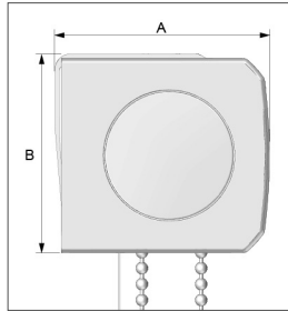
Dimensions A: 72 mm, B: 68 mm.
