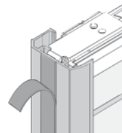
(A1) U-list med tape og vinkel. Til modell 3242 fås en kort vinkel, hvorpå wirefoot monteres. Sidelisten kan også monteres på glass.
