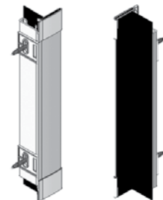
(A1) U-list med tape og vinkel. Til modell 3242 fås en kort vinkel, hvorpå wirefoot monteres. Sidelisten kan også monteres på glass.
