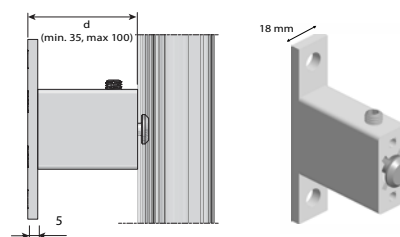
Avstandsbeslag, aluminium - 35-100 mm veggavstand
