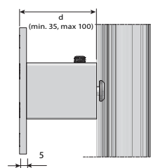
Avstandsbeslag, aluminium - 35-100 mm veggavstand
