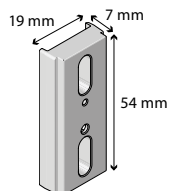
Afstandsstykke, 7 mm 50/70 mm
