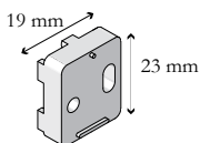
Afstandsstykke, 10 mm 16/25 mm
