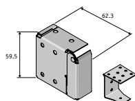
Endebeslag 50/70 mm incl U-beslag til midtplacering.
