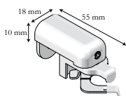
Beslag til plastvindue 16/25 mm.
